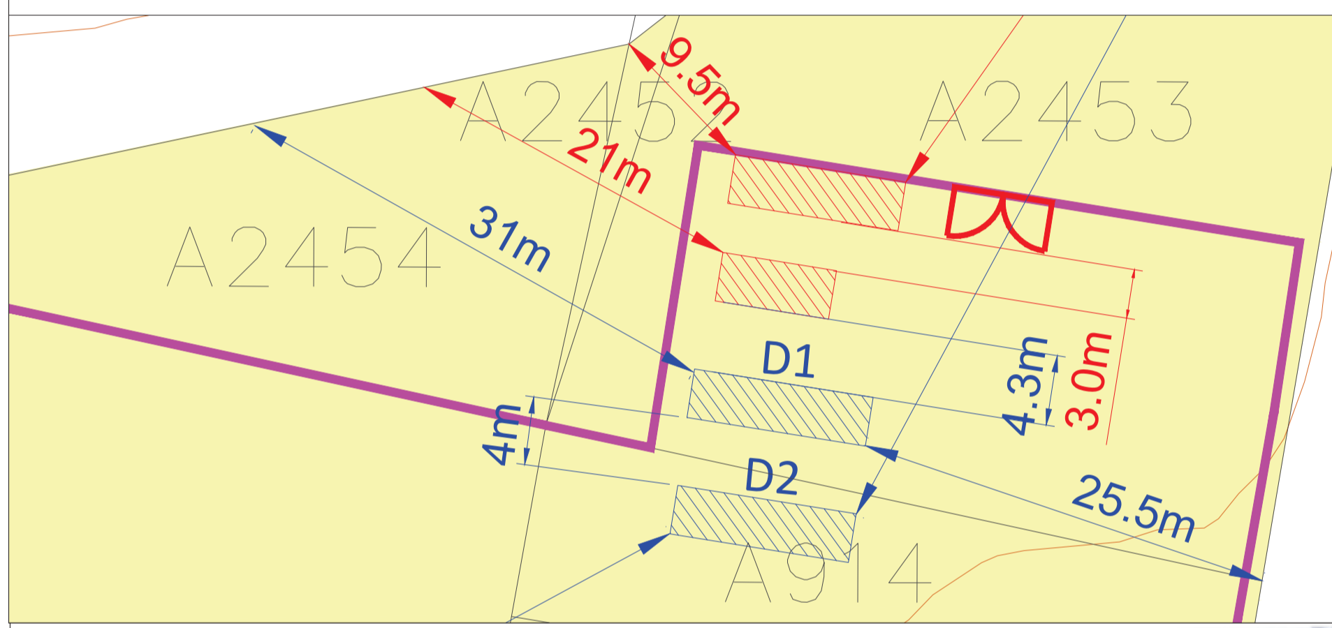
Sous-station de distribution (Echelle 1/100)
