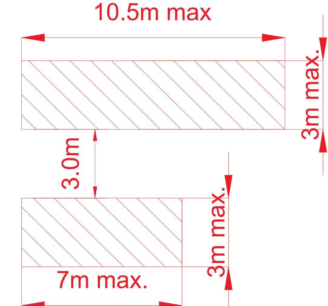
Structure de livraison (Echelle 1/100)
